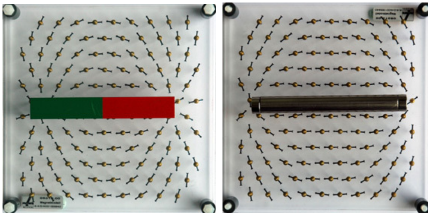
Abb. 4a und b: Magnetfeldlinien eines einfachen üblichen und eines selbst hergestellten Stabmagneten
