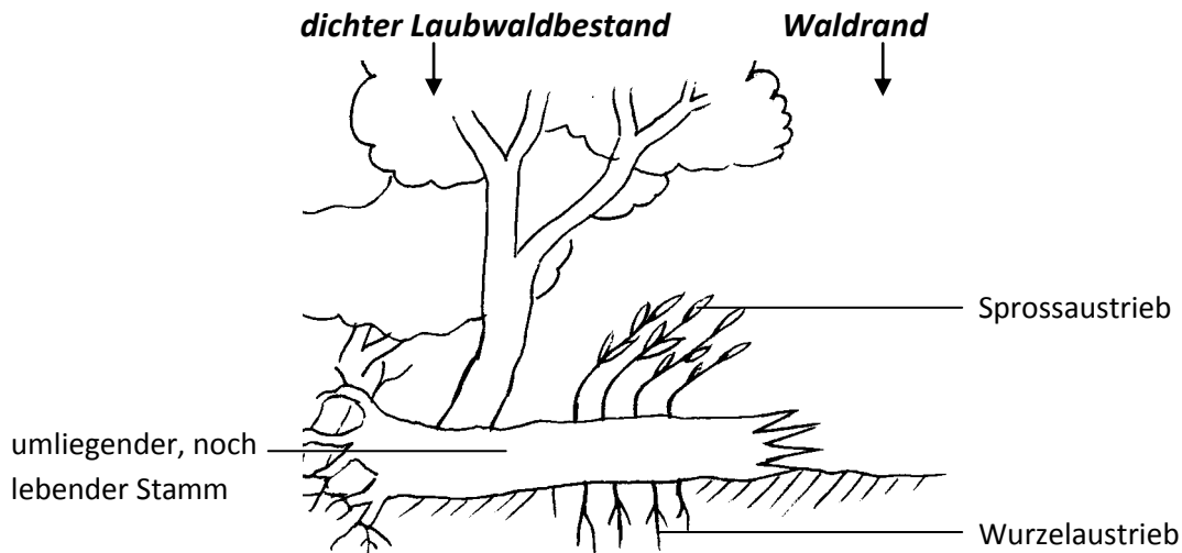
Abb.: Schematische Darstellung des Spross- und Wurzelaustriebs eines durch Sturm umgebrochenen, noch lebenden Laubbaumstammes. Grafik: F. KÖRNER
