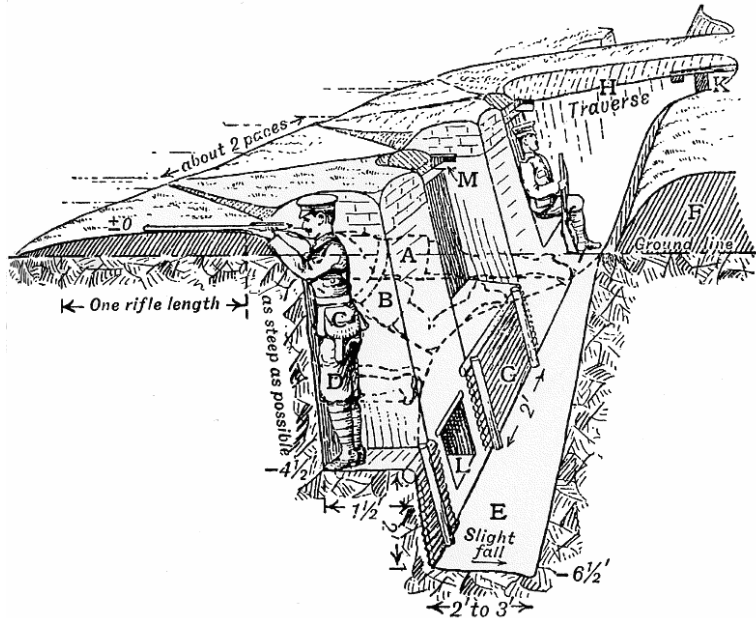
Grafik 1 | Britische Konstruktionszeichnung | 1914
